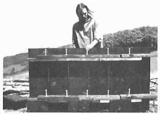
FIGURE 97 : BANCHE ARTICULEE PERMETTANT DES MURS COURBES AINSI QUE DES POTEAUX - POSITION RECTILIGNE (LE PIN, 1975)
