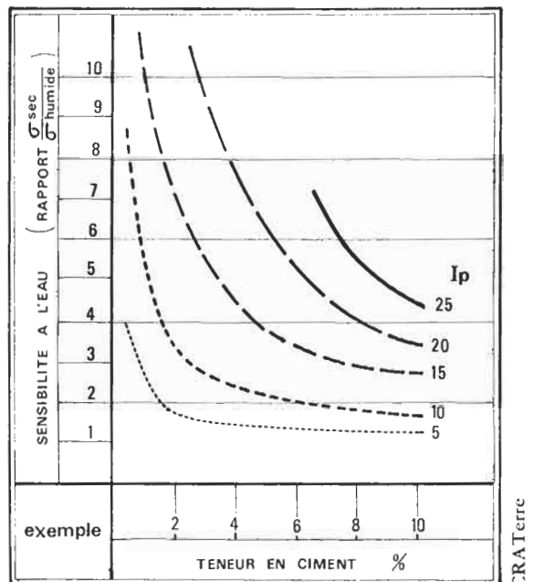
FIGURE 285 : SENSIBILITE A L'EAU SELON LA TENEUR EN CIMENT ET I_p POUR UN MEME COMPACTAGE
