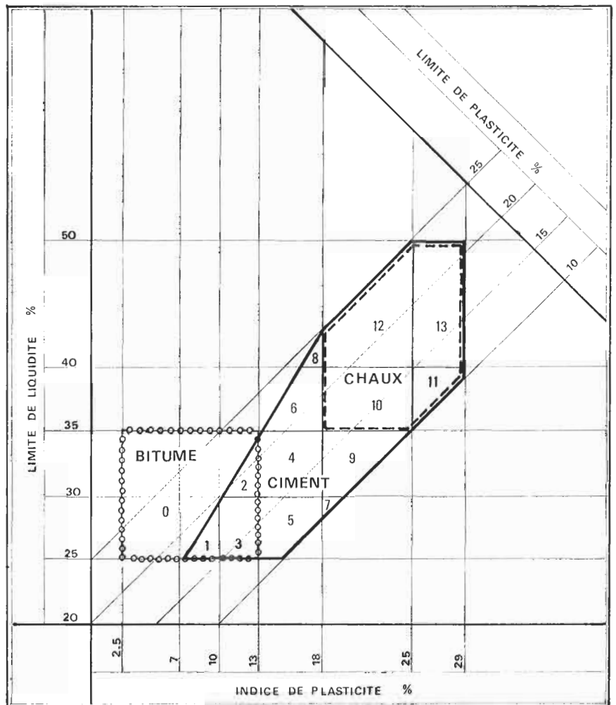
▲ FIGURE 281 : FUSEAU DE STABILISATION POUR LE CIMENT, LA CHAUX, LE BITUME, SEULS LES ÉLÉMENTS FINS (INFÉRIEURS À 0,5 mm) SONT PRIS EN CONSIDÉRATION
