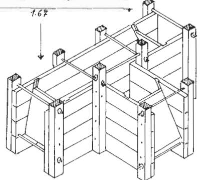
Banche pour mur de refend
