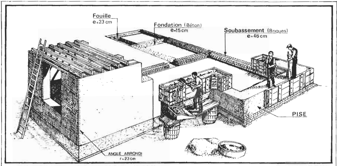
FIGURE 64 : ELEVATION D'UNE MAISON EN PISE EN GRANDE-BRETAGNE
