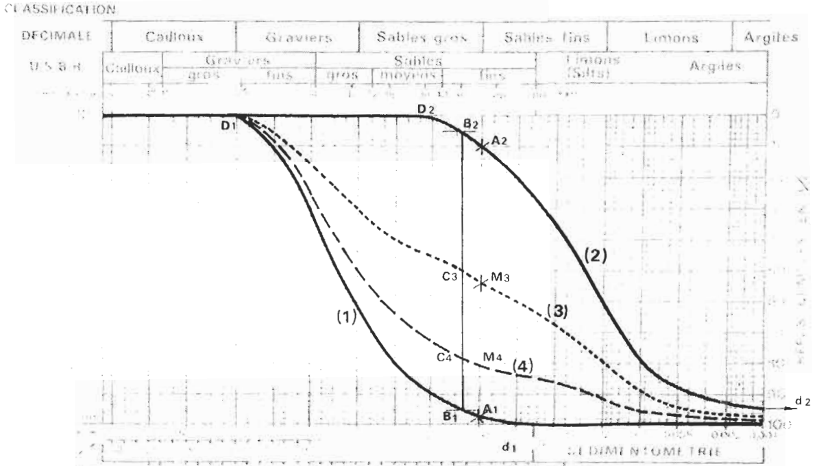
FIGURE 279 : DETERMINATION DE LA COURBE DE MELANGE DE DEUX SOLS. - EN TRAIT PLEIN : LES DEUX SOLS DE DEPART - EN TRAIT POINTILLE : LES MELANGES
