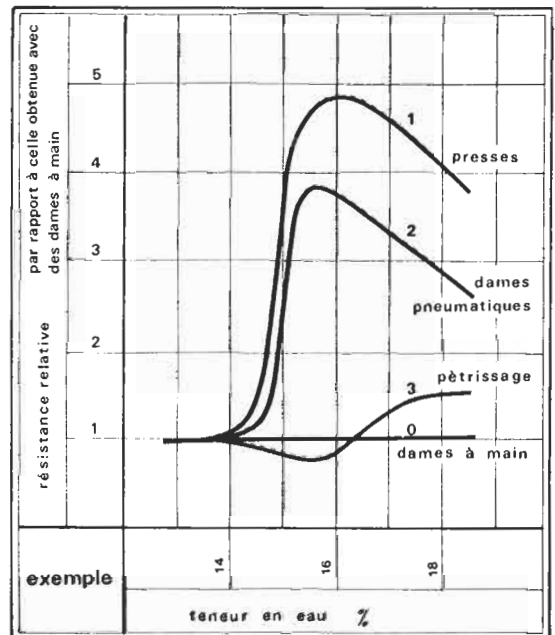
FIGURE 278 : RESISTANCES POUR UNE DEFORMATION DE L'ECHANTILLON DE 5%
