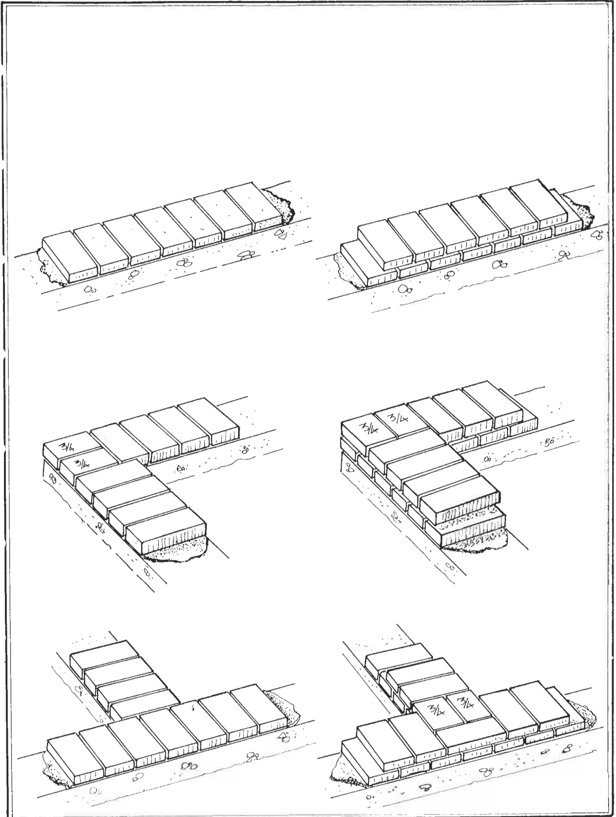
FIGURE 180 : APPAREILLAGES DE BRIQUES RECTANGULAIRES
