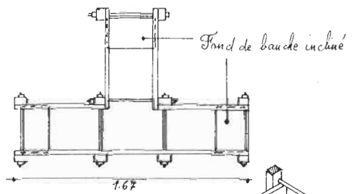
Banche roulante
