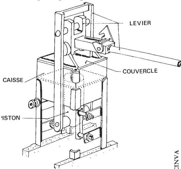
FIGURE 219 : LA PRESSE CINVA-RAM
