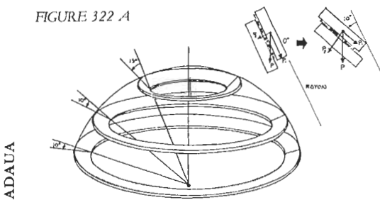
FIGURES 322 : PRINCIPE DE CONSTRUCTION DES COUPOLES SANS COFFRAGE
