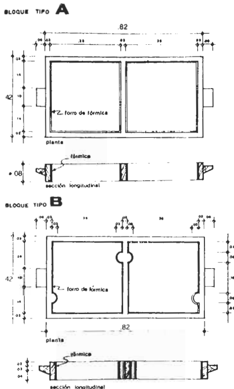
FIGURE 203 : MOULES UTILISÉS À CAYALTI
