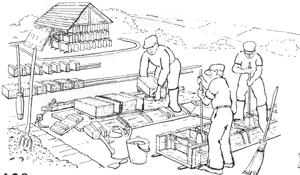
FIGURE 213 : BRIQUES DE TERRE DAMEE A LA MAIN EN R.D.A.
