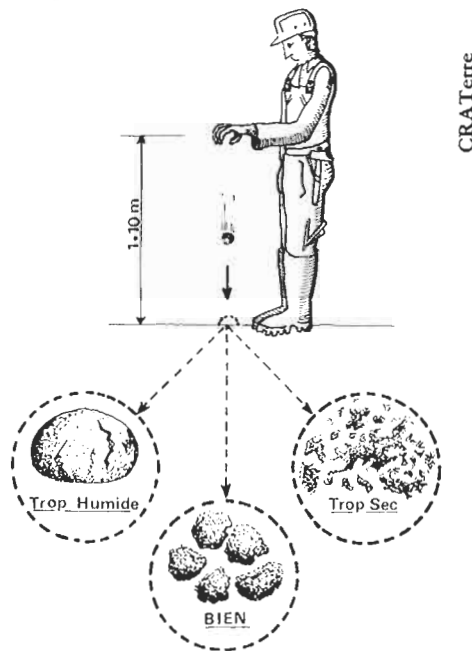
FIGURE 259 : VERIFICATION DE LA TENEUR EN EAU SUR CHANTIER
