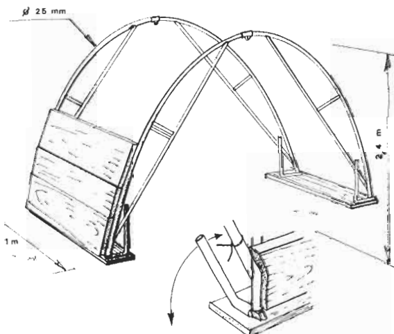
FIGURE 306 : COFFRAGE EXPERIMENTAL AVEC CAME FACILITANT LE DECOFFRAGE
