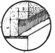
Detail de la feuillure "larmier"
