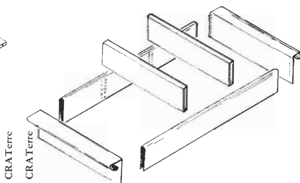
FIGURE 163 : 2 - MOULE EN TOLE POUR TROIS BLOCS DE 19 × 39 × 9 cm
