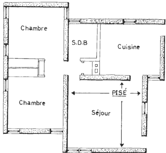
FIGURE 94 : EXEMPLE DE CONSTRUCTION ARCHITECTURALE ELIMINANT LES ANGLES EN PISÉ (HIBBEN)
