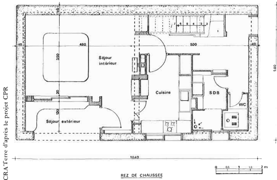
FIGURE 110 : REZ-DE-CHAUSSEE
