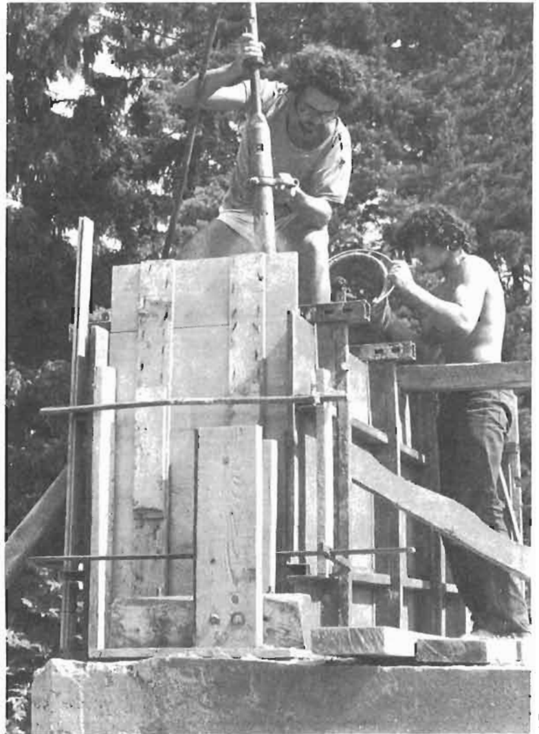
▲ FIGURE 96 : EXPERIENCE DU GROUPE « PALAFITTE » DE L'UP D'ARCHITECTURE DE GRENOBLE EN 1975 AU PIN (ISERE) - CONSTRUCTION CIRCULAIRE EN PISE
