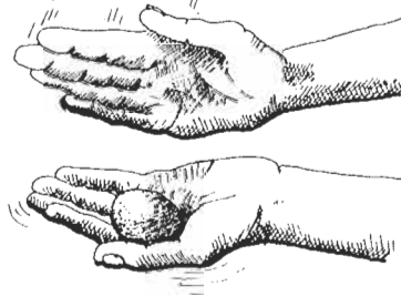
FIGURE 261 : ESSAI DE SECOUSSE
