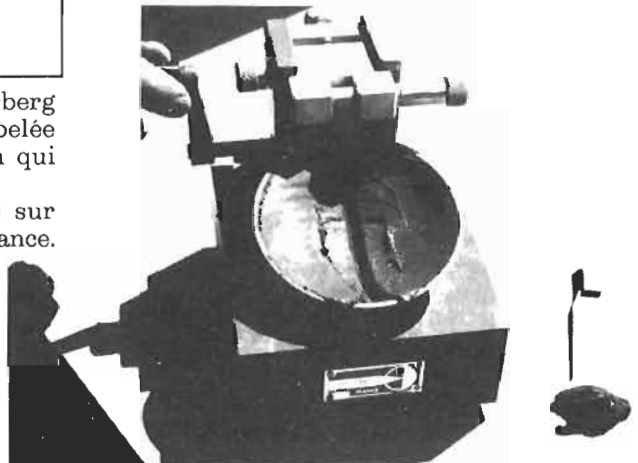
FIGURE 253 : APPAREIL DE CASAGRANDE POUR LES LIMITES D'ATTERBERG
