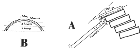
FIGURE 323 : CONSTRUCTION D'UNE COUPOLE SANS CINTRE
