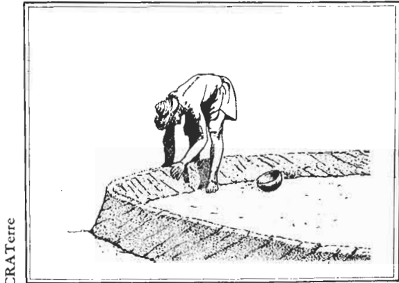
FIGURE 130 : LE MAÇON FAÇONNE A LA MAIN LA PREMIÈRE ASSISE
