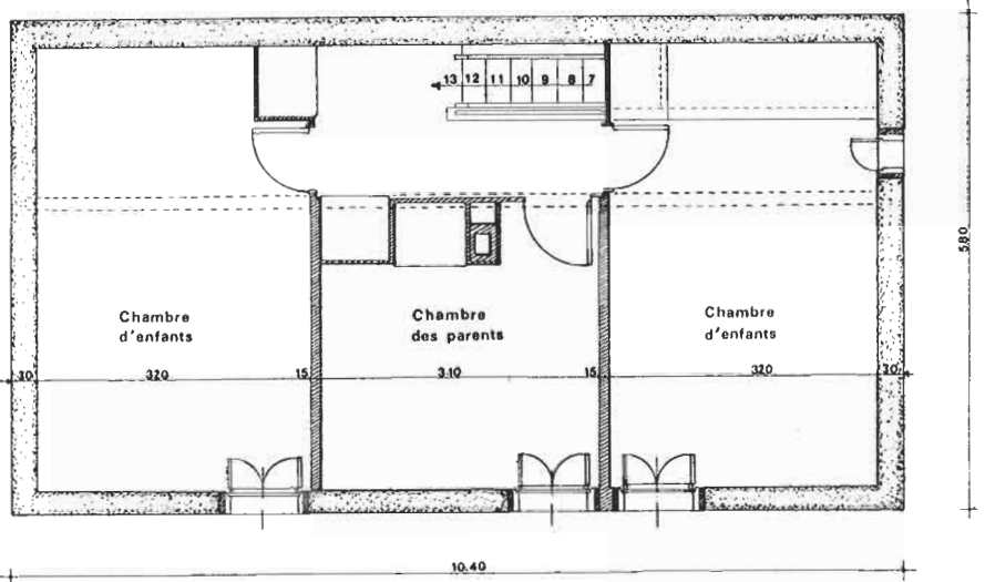
FIGURE 111 : ETAGE
