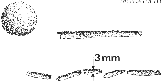
FIGURE 254 : DETERMINATION DE LA LIMITE DE PLASTICITE
