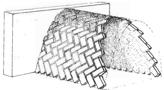
FIGURE 307 : APPAREILLAGE EN EPIS (OU EN CHEVRON)
