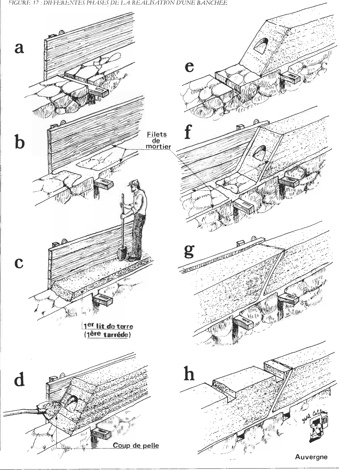
FIGURE 17 : DIFFERENTES PHASES DE LA REALISATION D'UNE BANCHEE
