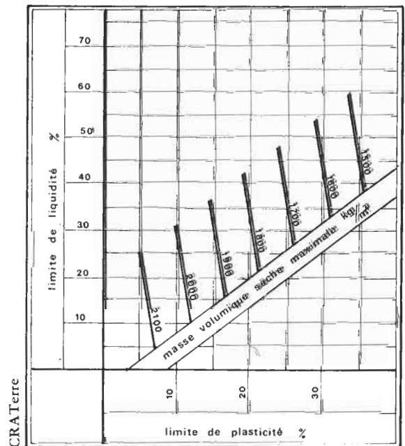
FIGURE 273 : LIMITES D'ATTERBERG ET DENSITE
