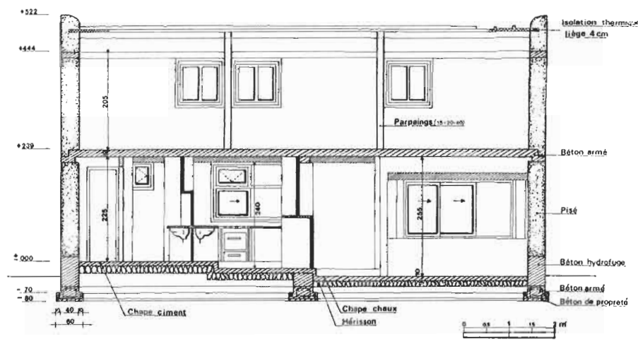
FIGURE 113 : COUPE LONGITUDINALE
