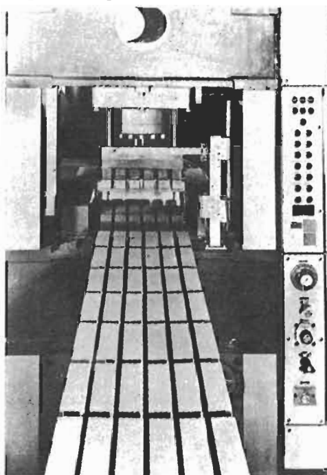
Figure 234 : presse Drostholm L3
