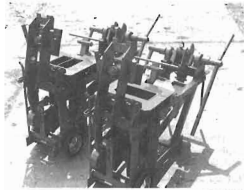
FIGURE 229 : PRESSE TERSTARAM. LA CHAÎNE EN S'ENROULANT AUTOUR DE L'ARBRE, FAIT REMONTER LE LEVIER QUI AGIT SUR LE PISTON.
