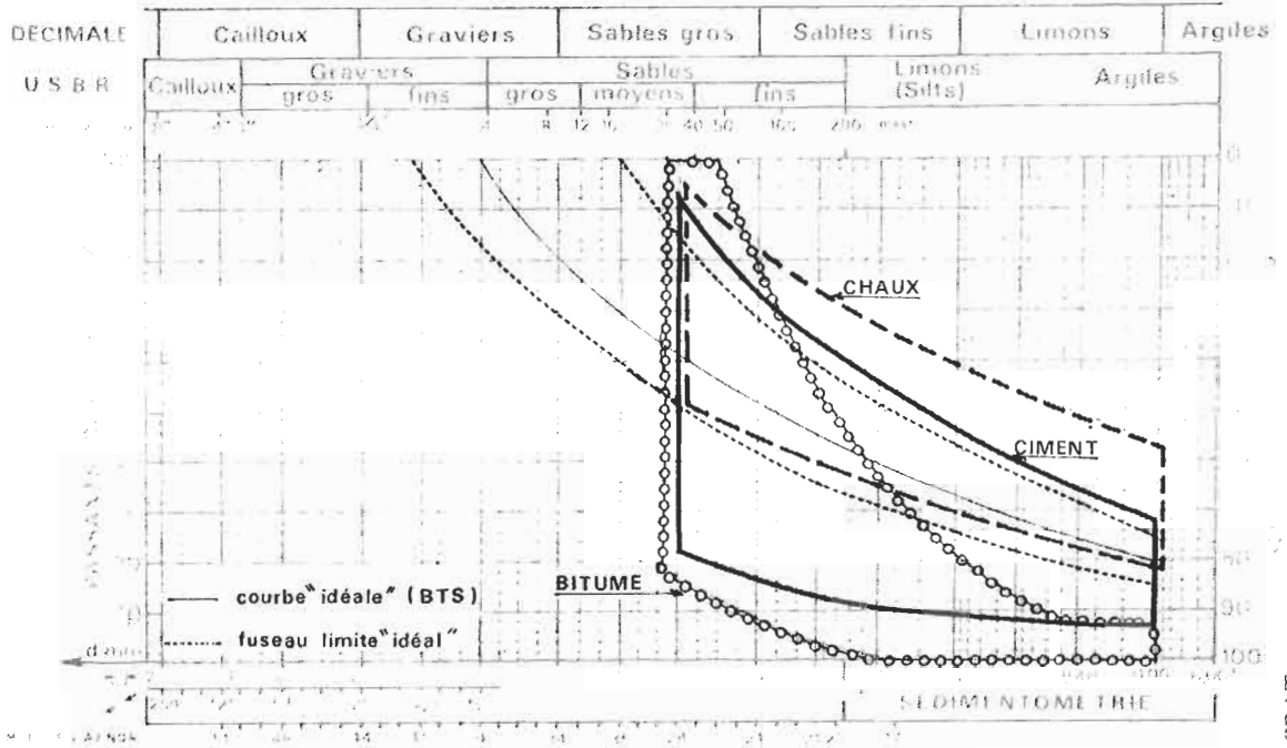
▲ FIGURE 281 : FUSEAU DE STABILISATION POUR LE CIMENT, LA CHAUX, LE BITUME, SEULS LES ÉLÉMENTS FINS (INFÉRIEURS À 0,5 mm) SONT PRIS EN CONSIDÉRATION
