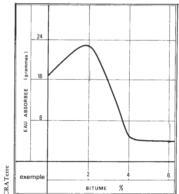
FIGURE 290 : ESSAI D'ABSORPTION
