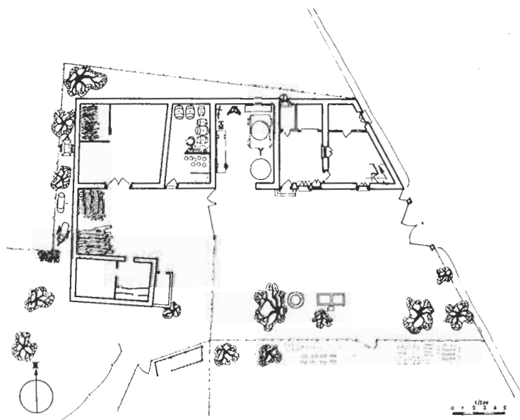
FIGURE 49 : PLAN D'ENSEMBLE
