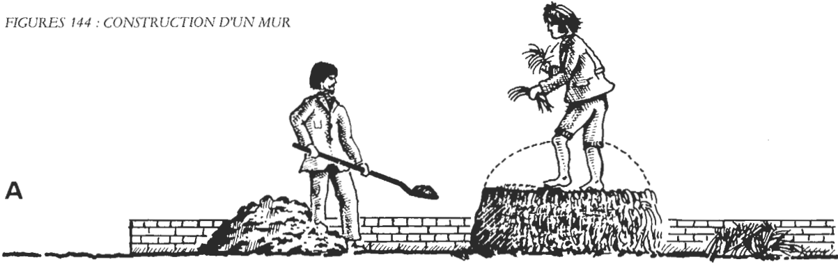
A : PREPARATION DU MELANGE : TERRE-PAILLE
