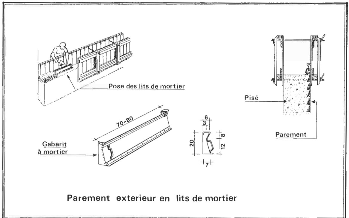
FIGURE 325 : PAREMENT EXTERIEUR EN LITS DE MORTIER
